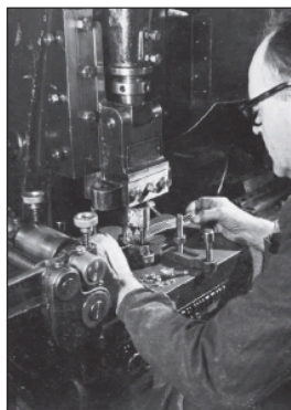
▼ Fig. 17 : Découpe d'un bracelet à la presse.
